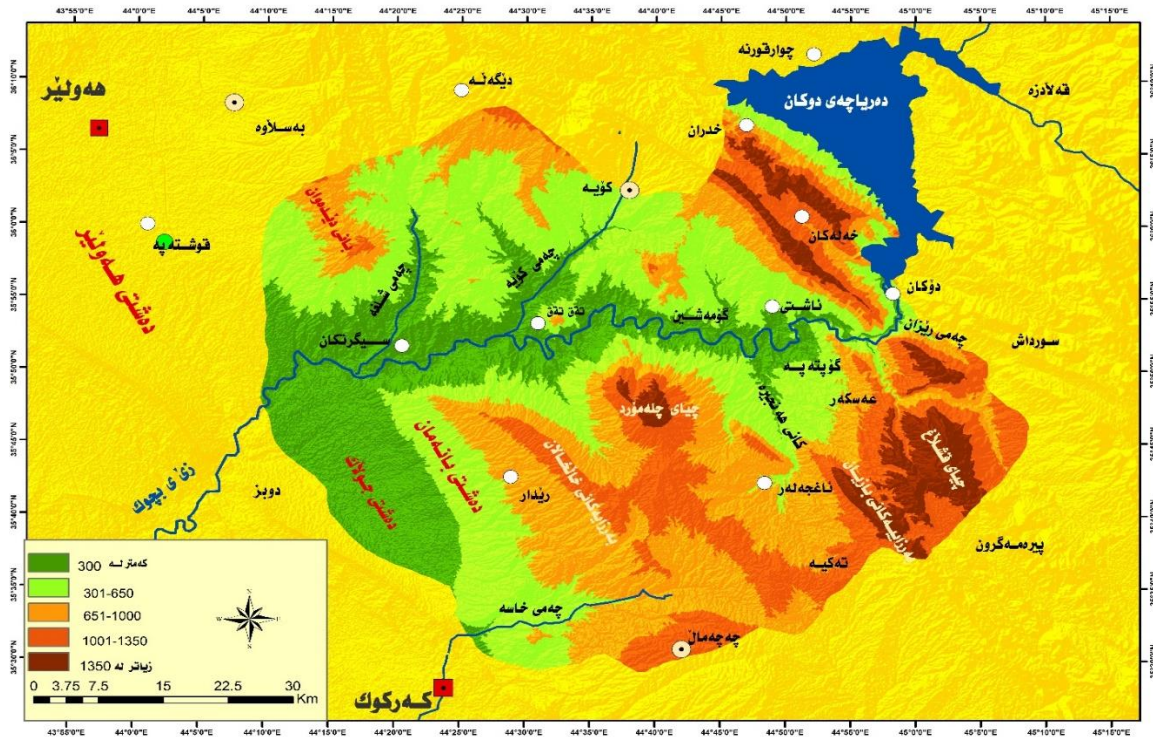
نه خسه ئی (3) به رزی و نزمی ئهو ناوچانه ئی بهر شالووی نه نفالی چوار کهوتن کاری توێژەر به به کار هینانی ArcGIS v.10,3 بارانی سالانه گه پشتر ته (346 - 451 - 479) ملم، خسته ئی (3).
